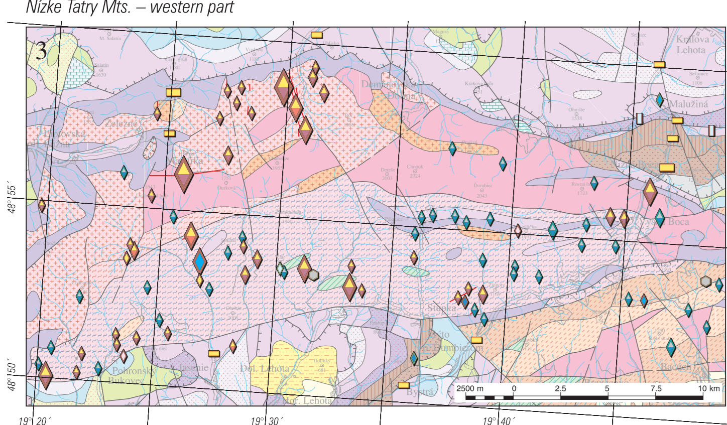
Nízke Tatry – západná časť Nízke Tatry Mts. – western part
