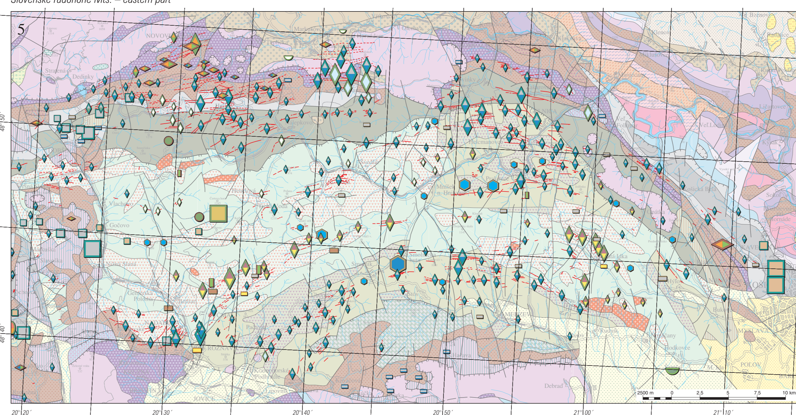
Slovenské rudohorie – východná časť Slovenské rudohorie Mts. – eastern part
