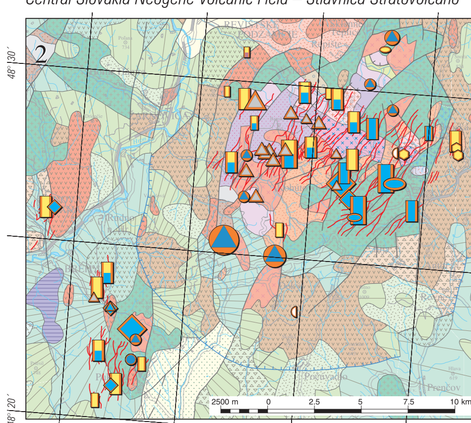
Stredoslovenské neovulkanity – Štiavnický stratovulkán Central Slovakia Neogene Volcanic Field – Štiavnica Stratovolcano
