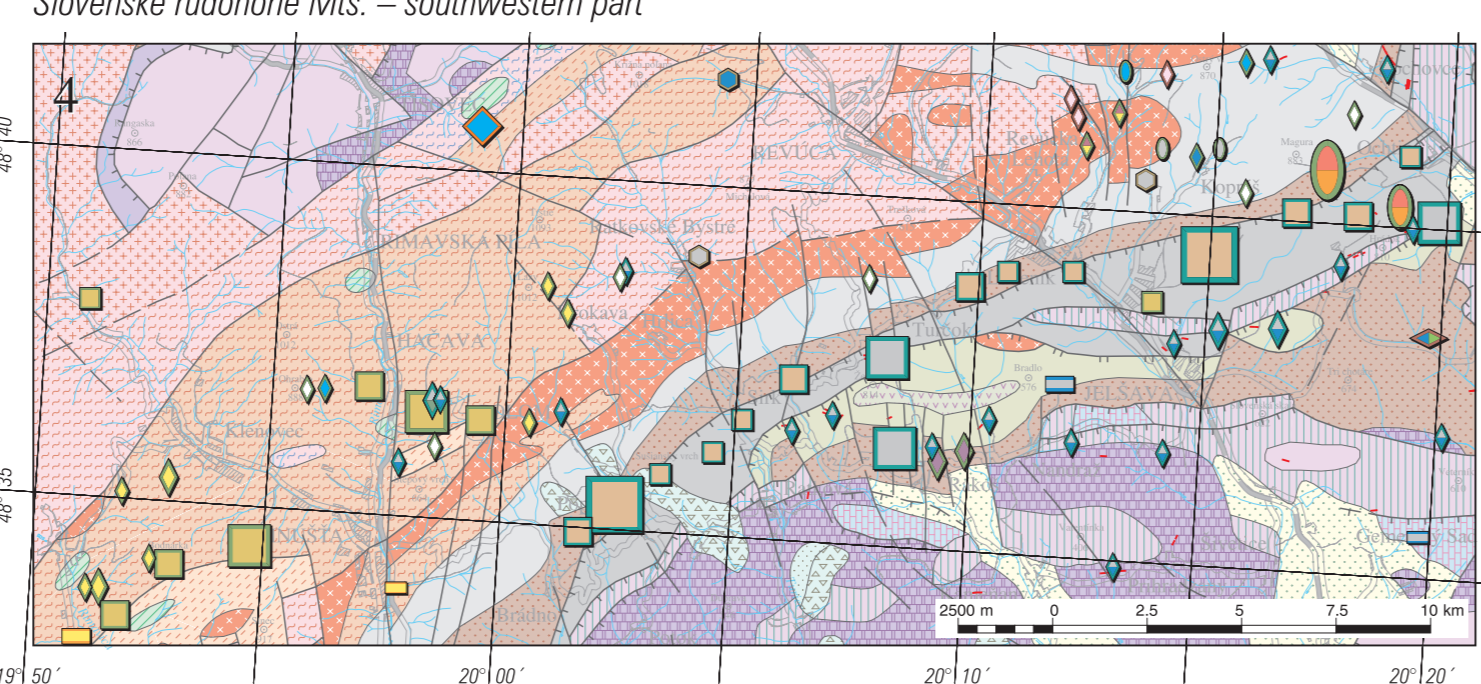
Slovenské rudohorie – juhozápadná časť Slovenské rudohorie Mts. – southwest part
