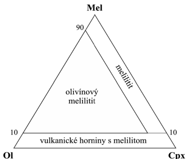
Obr. 3. Modálna klasifikácia vulkanických hornín s obsahom melilitu (Streckeisen, 1978) založená na obsahu melilitu (Mel), olivínu (Ol) a klinopyroxénu (Cpx).
