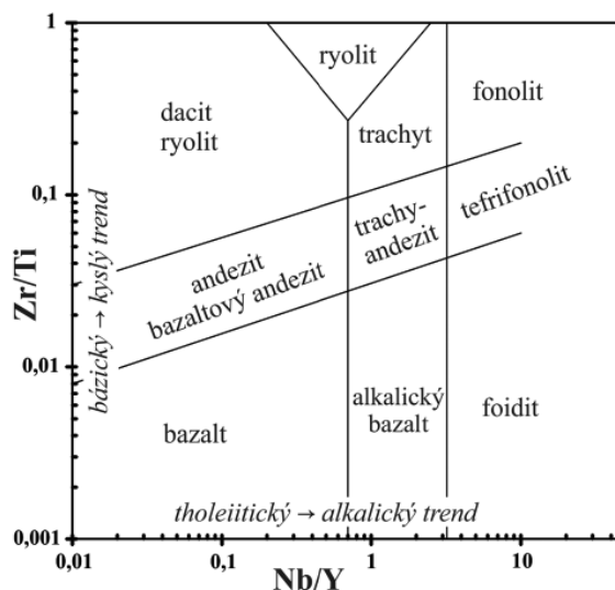
Obr. 11. Proxy TAS diagram nemobilných prvkov (upravené podľa Pearce, 1996, 2014, a Floyd a Winchester, 1975).
