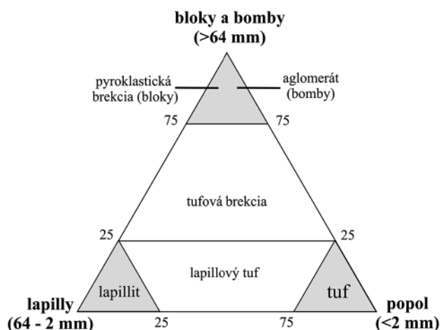
Obr. 1. Klasifikácia polymodálnych pyroklastických (vulkano-klastických) hornín na základe proporcionálneho zastúpenia pyroklastov rôznej veľkosti (Fisher, 1966).
