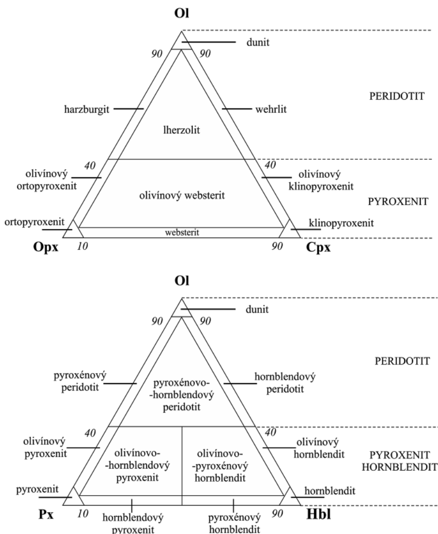
Obr. 6. Modálna klasifikácia ultramafických hornín založená na obsahu olivínu (Ol), ortopyroxénu (Opx), klinopyroxénu (Cpx), pyroxénu (Px) a hornblendu (Hbl) podľa Streckeisen (1973).
