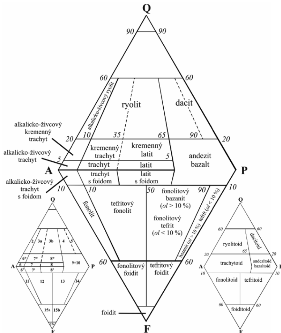
Obr. 7. Modálna QAPF klasifikácia vulkanických hornín (Streckeisen, 1978). Vrcholy dvojitého trojuholníka sú: Q = kremeň; A = alkalický živec; P = plagioklas a F = foid. Nesmie sa použiť na klasifikáciu hornín, v ktorých je obsah mafických minerálov M > 90 %.
