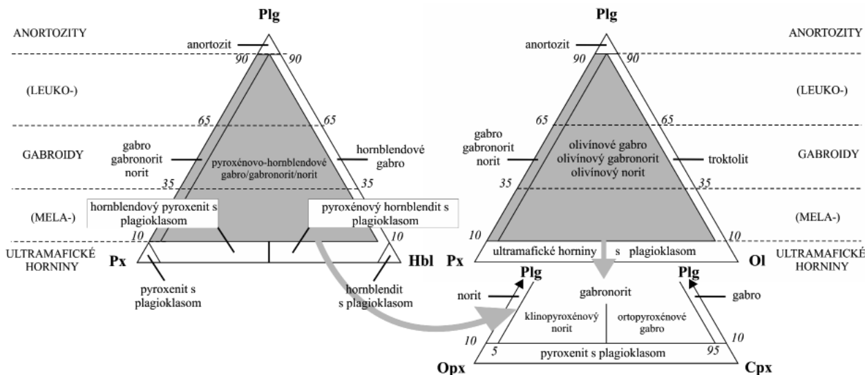
Obr. 5. Modálna klasifikácia gabroidných hornín založená na obsahu plagioklasu (Plg), pyroxénu (Px), olivínu (Ol), ortopyroxénu (Opx), klinopyroxénu (Cpx) a hornblendu (Hbl) podľa Streckeisen (1976). Horniny spadajúce do sivých trojuholníkových polí v klasifikačných diagramoch môžu byť ďalej rozdelené v klasifikačnom diagrame, ku ktorému smerujú šípky.
