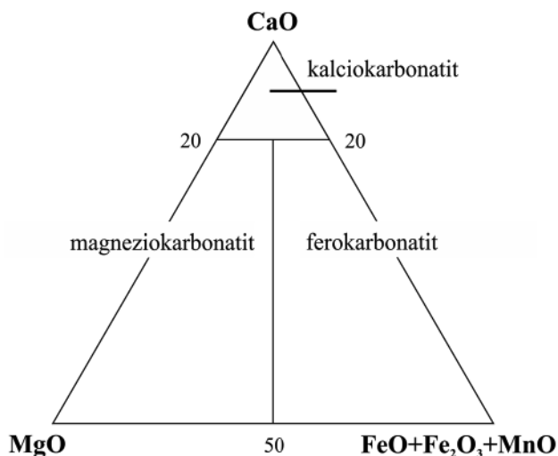
Obr. 2. Chemická klasifikácia karbonatitov založená na hmot. % oxidov (Wooley a Kempe, 1989). Používa sa pre karbonatity s obsahom \text{SiO}_2 < 20\% . Karbonatity s obsahom \text{SiO}_2 > 20\% sú silikokarbonatity .
