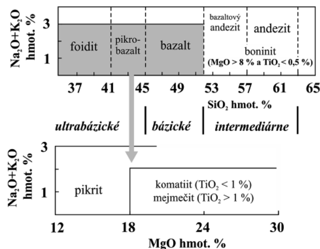
Obr. 9. Chemická klasifikácia a odlíšenie „vysokohorečnatých“ vulkanických hornín, boninitu, mejmečitu, komatiitu a pikritu (Le Bas, 2000). Ak hornina spadá do šedého poľa v TAS diagrame (horný diagram) a má zvýšený obsah MgO, treba skontrolovať, či nejde o komatiit, mejmečit a pikrit, a to skôr, ako sa pomenuje foidit, pikrobazalt alebo bazalt. Obdobne, ak má hornina viac ako 52 hmot. % SiO_2 , treba skontrolovať, či spĺňa kritériá na klasifikáciu boninitu.
