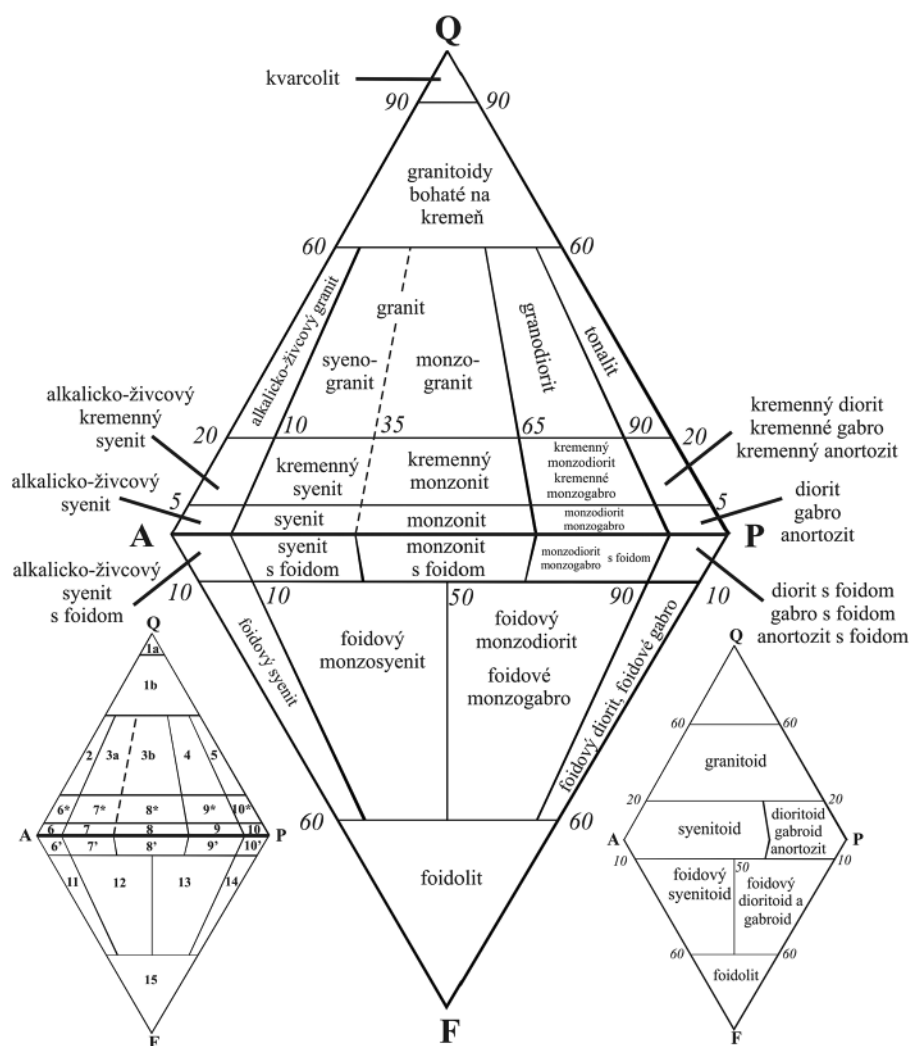
Obr. 4. QAPF modálna klasifikácia plutonických hornín podľa Streckeisen (1976). Vrcholy dvojitého trojuholníka sú Q = kremeň, A = alkalický živec, P = plagioklas a F = foidy (feldšpatoidy). Diagram sa nesmie používať pri horninách, ktoré majú obsah mafických minerálov väčší ako 90 %. Malá schéma vľavo je QAPF diagram s označenými poľami (Streckeisen, 1976). Poľa 6* až 10* sú presýtené Si a poľa 6' až 10' sú nedosýtené Si varianty poľí 6 až 10. Malá schéma vpravo je predbežná QAPF klasifikácia plutonických hornín na terénne použitie podľa Streckeisen (1976).
