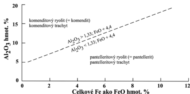
Obr. 10. Klasifikácia trachytov a ryolitov do komenditového a pantelleritového typu na základe obsahu \text{Al}_2\text{O}_3 a celkového obsahu Fe ako FeO (MacDonald, 1974). Koordináty ľavého spodného okraja čiary sú 0,45 a 5,0 a pravého horného okraja 10,98 a 19,0.
