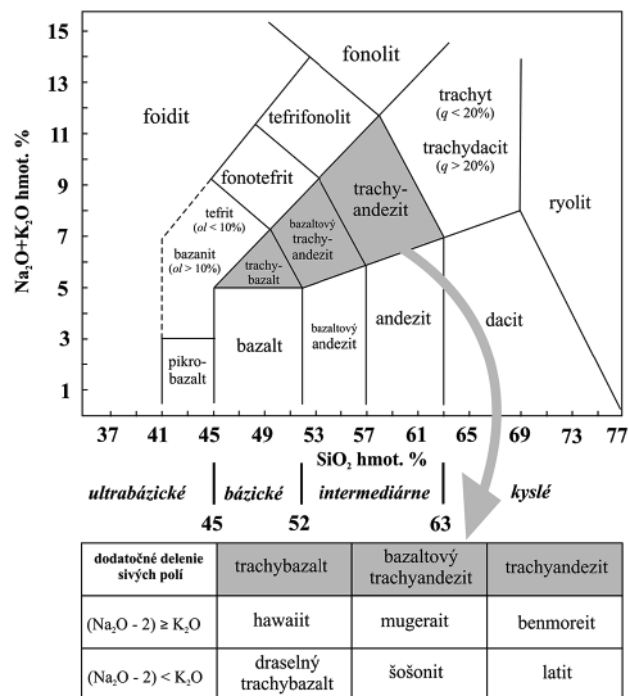
Obr. 8. Chemická klasifikácia vulkanických hornín založená na celkovom obsahu alkálií ( Na_2O + K_2O hmot. %) a obsahu SiO_2 (hmot. %) – (Le Bas et al., 1986). Horniny spadajúce do sivého poľa sa ďalej bližšie klasifikujú podľa tabuľky, ku ktorej smeruje šípka. Línia medzi polom foiditu a bazanitu a tefritu je čiarkovaná, lebo sú potrebné ďalšie kritériá na oddelenie týchto horninových typov. Značky: ol = normatívny olivín; q = normatívny 100 * Q / (Q + or + ab + an) .
