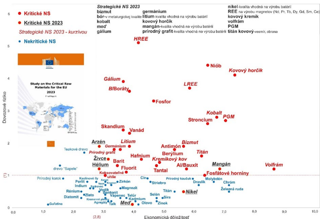
Rozdelenie sledovaných kovov a nerastných surovín z pohľadu posledného hodnotenia, správa európskej komisie stav k marcu 2023; upravené podľa European Commission, 2023
