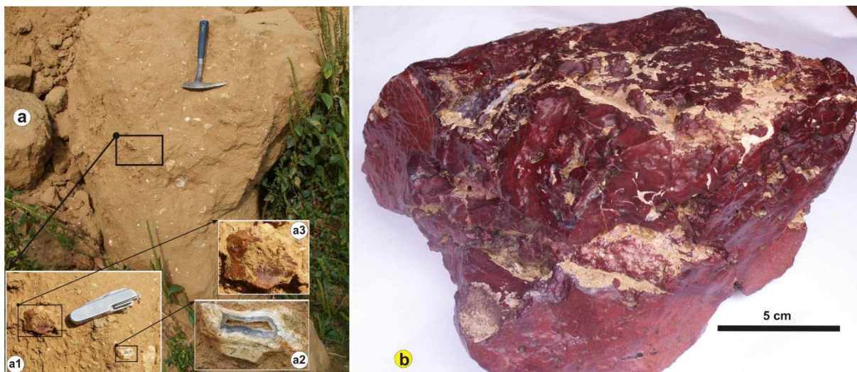
Zo steny uvoľnený blok čiastočne spevneného piesku (a) s vrstvou obsahujúcou úlomky hornín z podložného extruzívneho telesa (úlomky opálov, jaspisov - a1, 3 a chalcedónu s achátovou textúrou – a2). Úlomky hornín sú intenzívne obrúsené („tromblované“) pieskom navievaným vetrom. Zvlášť zreteľné je zaoblenie inak ostrých hrán úlomkov opálov a jaspisov (b). Foto: Z. Kollová a-a1, a2, a3; P. Bačo (b).
