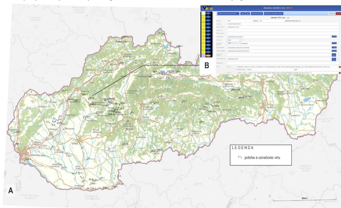
Mapa spracovaných hlbokých vrtov do databázy. B – Příklad náhledu metráže vo vrte DB-15 (Horný) v aplikácii databázy vrtov.
