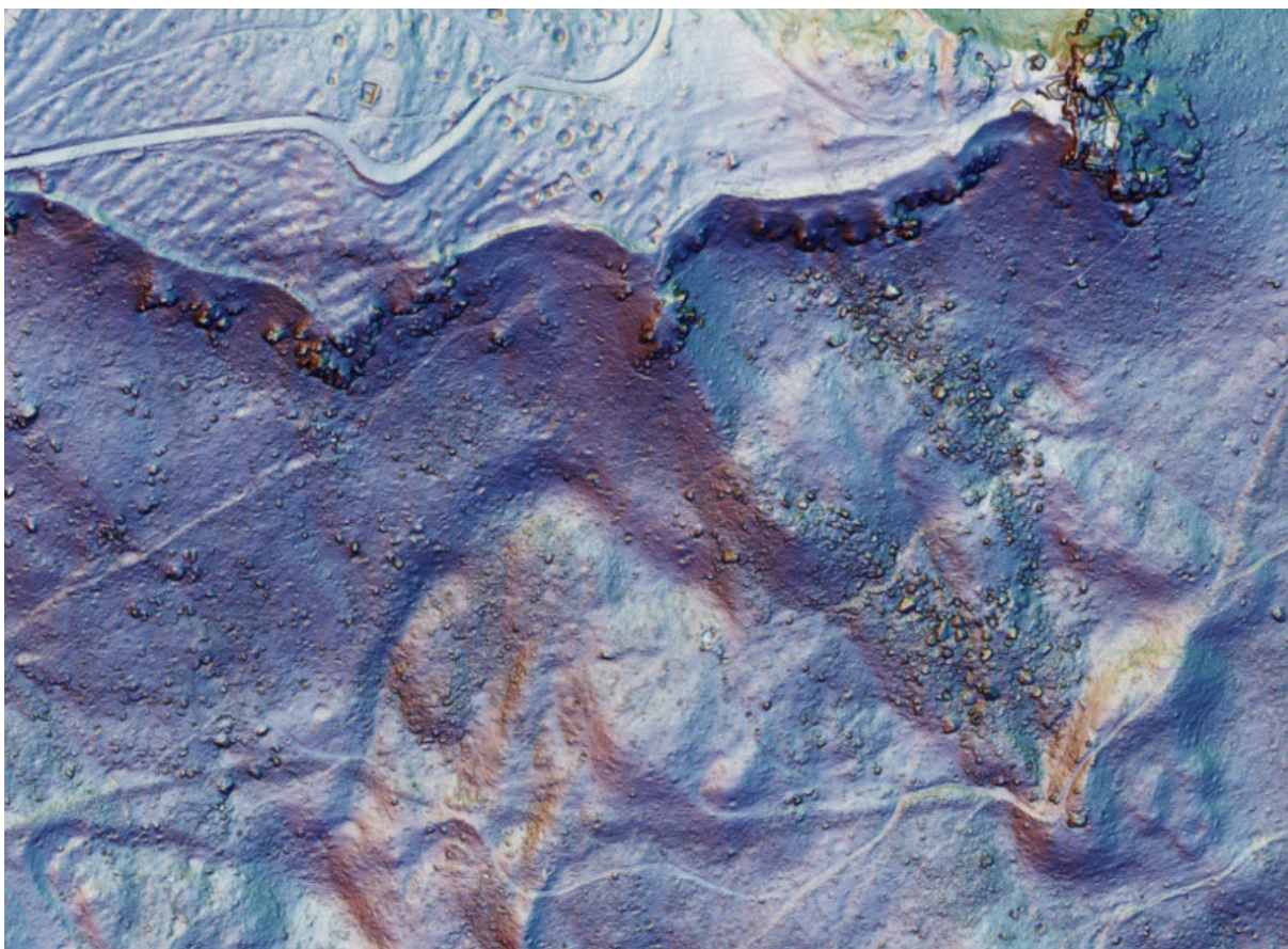
Ukážka podrobného DMR 5.0: Skorušinské vrchy pri obci Oravský Biely Potok, okr. Tvrdošín – rozsiahle zosuvy vyvinuté v paleogéne podtatranskej skupiny vo flyšovom vývoji; zreteľná tiež výrazná vrstevnatosť pieskovcových vrstiev bielopotockého súvrstvia; 49.25178920, 19.54370132 (zdroj produktov LLS: ÚGKK SR, spracovanie DMR: Ing. Tibor Lieskovský, PhD.)
