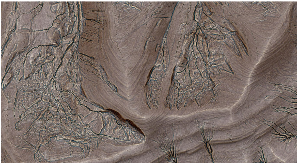
Ukážka podrobného DMR 5.0: Skorušinské vrchy pri obci Oravský Biely Potok, okr. Tvrdošín – rozsiahle zosuvy vyvinuté v paleogéne podtatranskej skupiny vo flyšovom vývoji; zreteľná tiež výrazná vrstevnatosť pieskovcových vrstiev bielopotockého súvrstvia; 49.25178920, 19.54370132 (zdroj produktov LLS: ÚGKK SR, spracovanie DMR: Ing. Tibor Lieskovský, PhD.)
