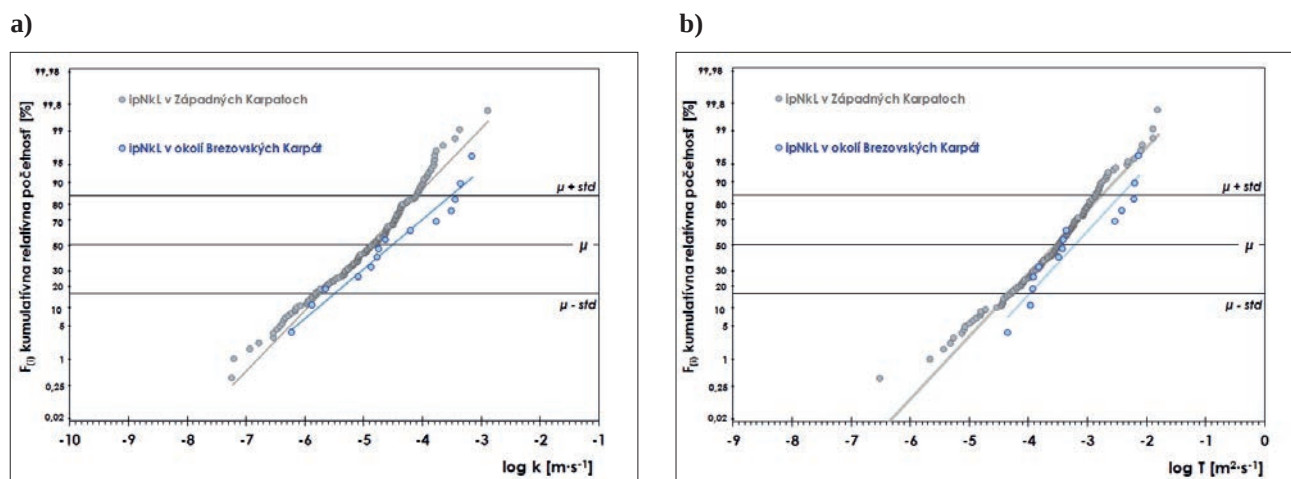
Obr. 14. Porovnanie štatistického rozdelenia hodnôt koeficientu filtrácie a koeficientu prietochnosti ílovcov, siltovcov, prachovcov, pieskovcov, pieskov a tufov v oboch súboroch prietrzských vrstiev z oblasti Brezovských Karpát a ich okolia a zo všetkých vrtov situovaných v analogických horninách v Západných Karpatoch: a) hodnoty koeficientu filtrácie, b) hodnoty koeficientu prietochnosti na kvantilových diagramoch.
