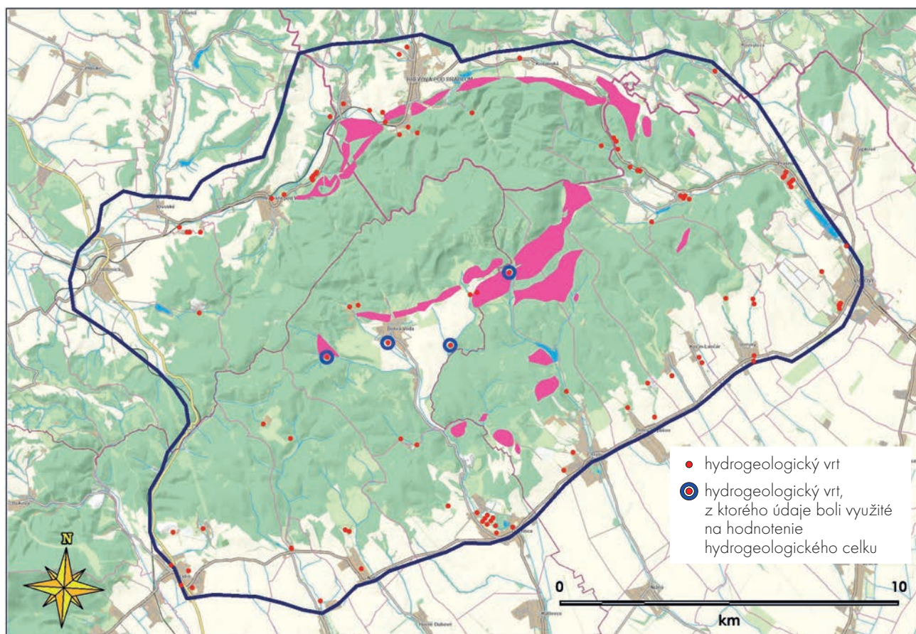
Obr. 15. Plošné rozšírenie hydrogeologického celku baraneckých pieskovcov, valchovských zlepencov a schizofytových vápencov brezovskej kriedy – karbonátových pieskovcov, polymiktých a brekciovitých zlepencov, piesčitých sliên a vápencov (pzsvK BR ) – na hodnotenom území Brezovských Karpát. Odkryté horniny celku sú znázornené purpurovou farbou, hranica územia má modrú farbu. Na území sú znázornené aj polohy hydrogeologických vrtov (bodové značky červenej farby).
