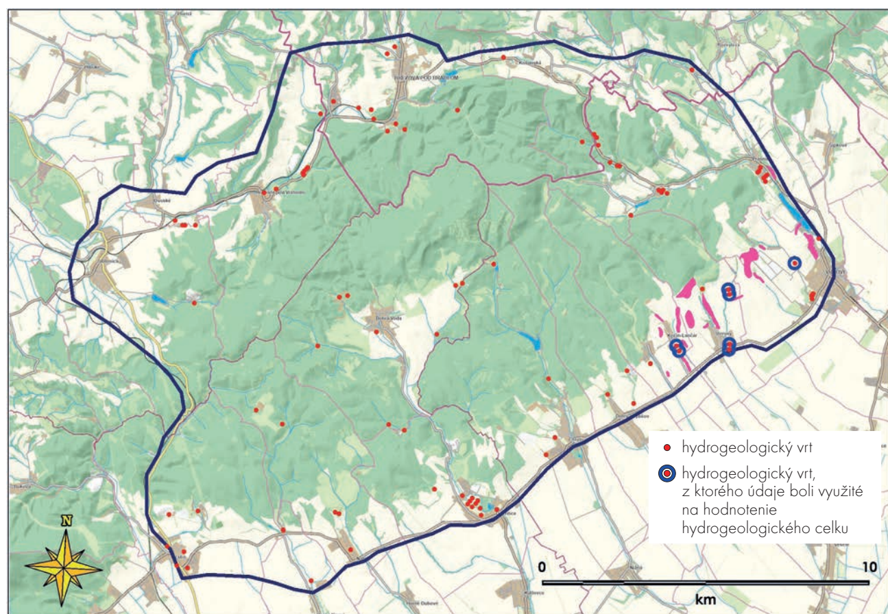
Obr. 19. Plošné rozšírenie hydrogeologického celku podbrančských pieskoviec a zlepcov lužického súvrstvia (egenburg – pN^{eLPB} ) na hodnotenom území Brezovských Karpát. Odkryté horniny celku sú znázornené purpurovou farbou, hranica územia má modrú farbu. Na území sú znázornené aj polohy hydrogeologických vrtov (bodové značky červenej farby).
