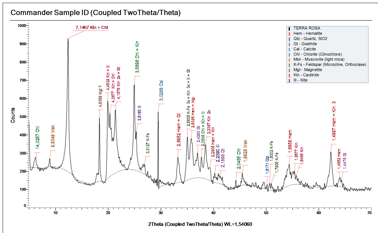
Fig. 9. XRD pattern of terra rossa.
